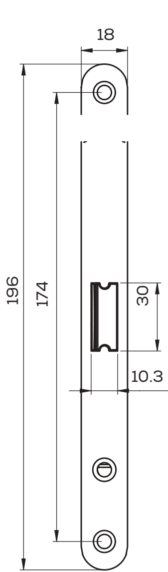
Gövde Tipi Case Type Kapalı Closed
