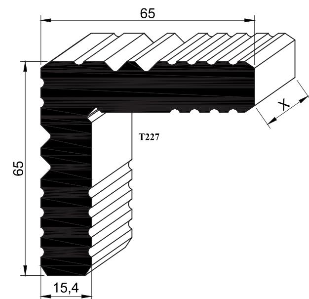
L501 - 4.509 kg/mt
