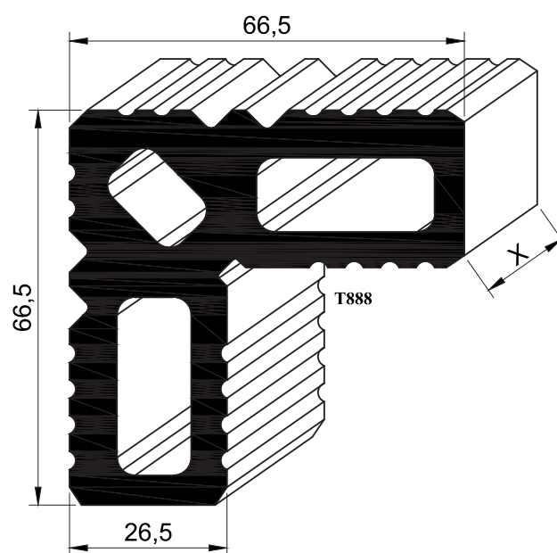
L503 - 4.921 kg/mt
