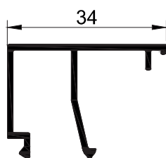
T75 - 0.300 kg/mt
