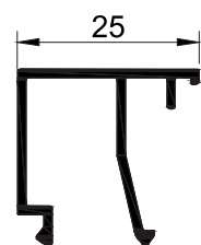
T275 - 0.268 kg/mt
