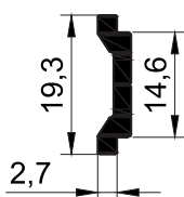
T225 - 0.164 kg/mt
