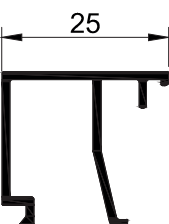
T275 - 0.270 kg/mt
