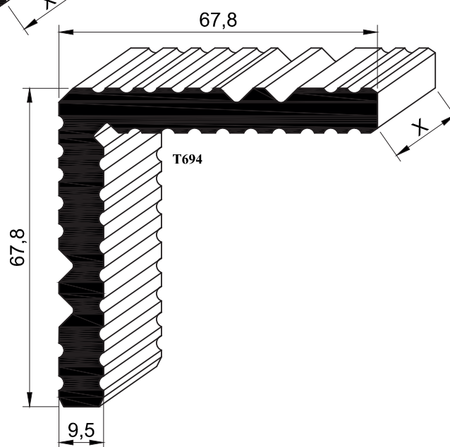
L505 - 2.886 kg/mt
