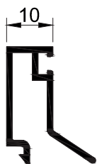
T1046 - 0.230 kg/mt
