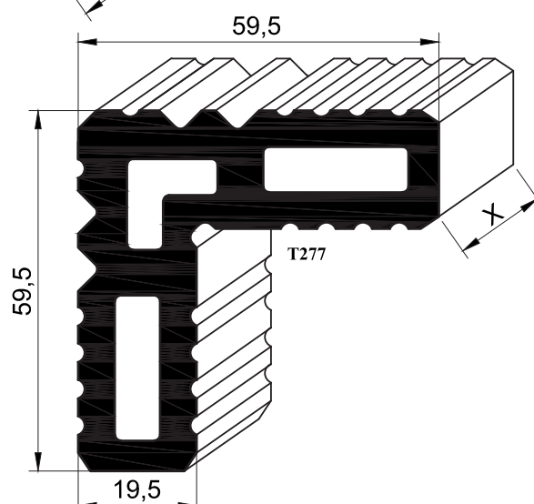
L504 - 3.622 kg/mt
