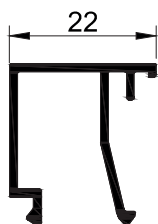
T276 - 0.259 kg/mt
