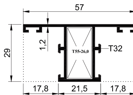
SZS67 T 08 - 0.560 kg/mt
