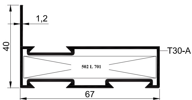
SZS67 T 07 - 0.728 kg/mt
