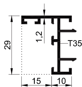
SZS67 T 03 - 0.330 kg/mt
