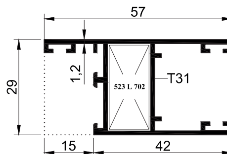
SZS67 T 02 - 0.650 kg/mt
