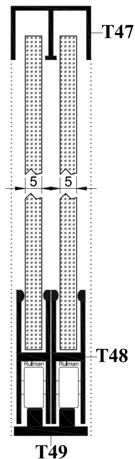
A -A Detayı
