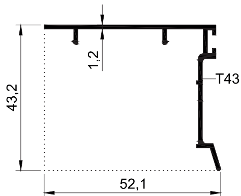
SZS100 T 04 - 0.435 kg/mt
