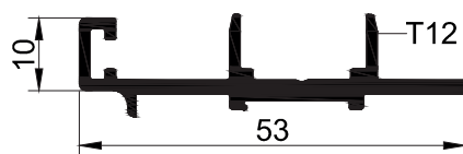
SZS100 T 08 - 0.497 kg/mt
