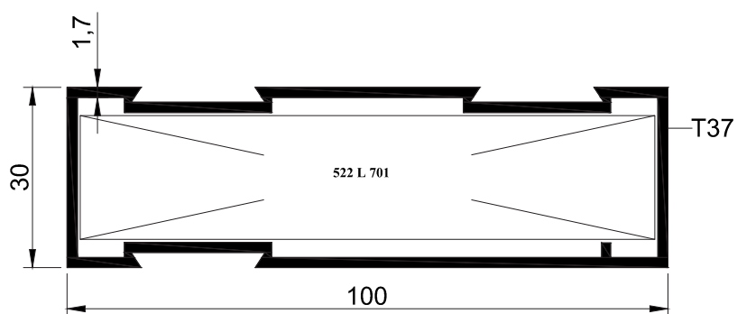
SZS100 T 01 - 1.260 kg/mt
