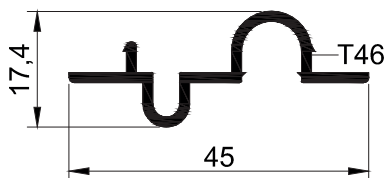
SZS100 T 05 - 0.313 kg/mt
