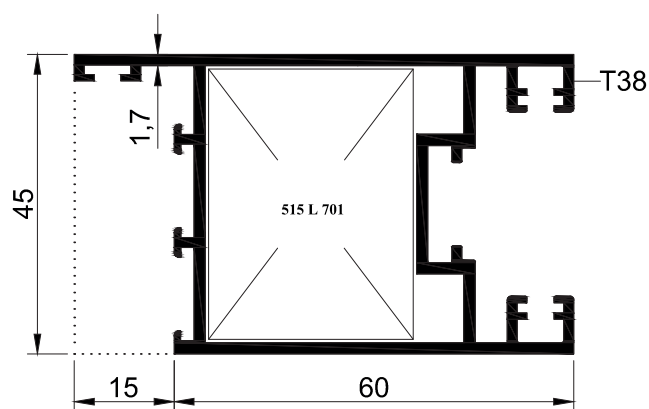
SZS100 T 02 - 1.320 kg/mt
