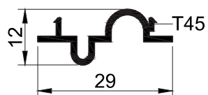
SZS67 T 05 - 0.177 kg/mt
