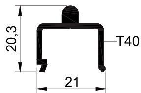
SZS100 T 06 - 0.270 kg/mt
