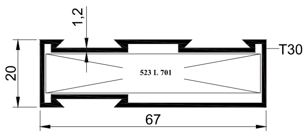
SZS67 T 01 - 0.660 kg/mt
