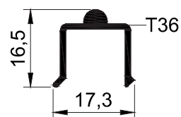
SZS67 T 06 - 0.170 kg/mt
