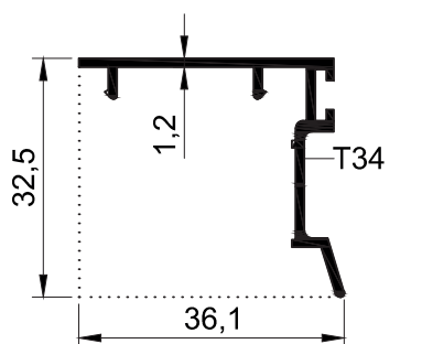
SZS67 T 04 - 0.290 kg/mt
