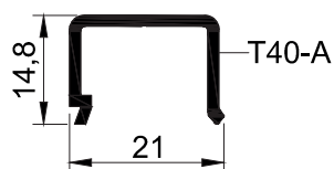
SZS100 T 07 - 0.192 kg/mt
