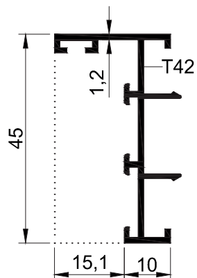
SZS100 T 03 - 0.390 kg/mt
