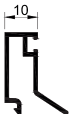
T1046 - 0.285 kg/mt
