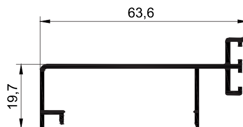
T572 - 0.765 kg/mt
