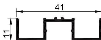
T2481 - 0.236 kg/mt
