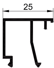
T275 - 0.270 kg/mt
