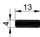
T463 - 0.137 kg/mt
