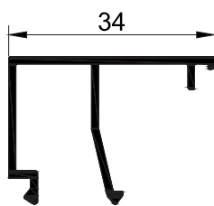
T75 - 0.300 kg/mt
