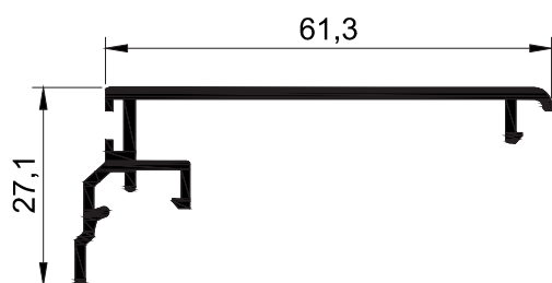
T2474-A - 0.490 kg/mt
