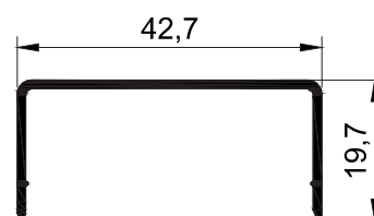
T2479 - 0.253 kg/mt
