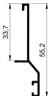
T2475 - 0.240 kg/mt
