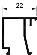
T276 - 0.259 kg/mt
