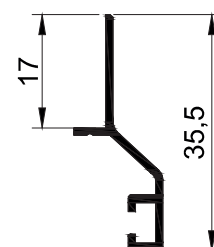
T2476 - 0.170 kg/mt
