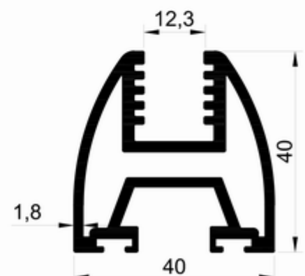
T 2161 - 1.182 kg/m
