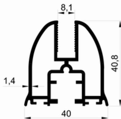
T 2426 - 0.860 kg/m
