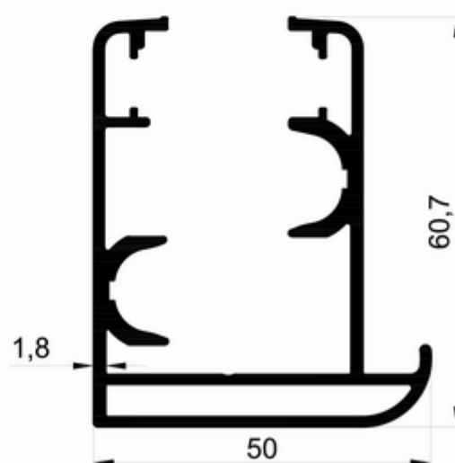
T2522 - 1.352 kg/m
