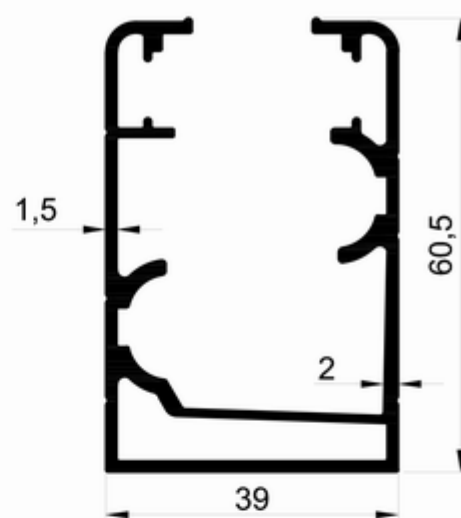
T 2415 - 1.100 kg/m
