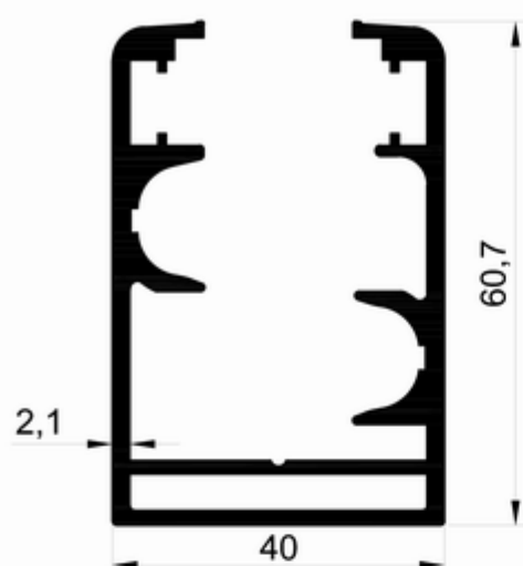
T 2515 - 1.465 kg/m
