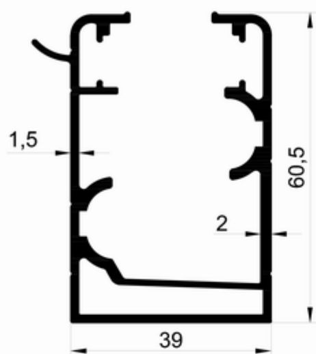
T 2414 - 1.140 kg/m
