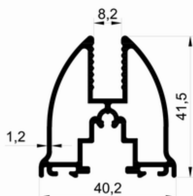
T 2416 0.820 kg/m
