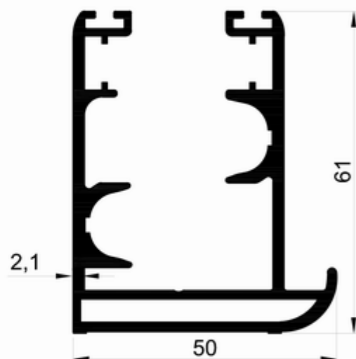
T1073-A - 1.810 kg/m
