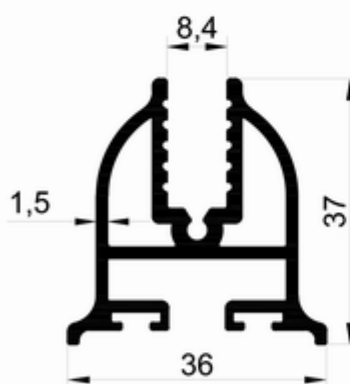
T 2290 - 0.810 kg/m
