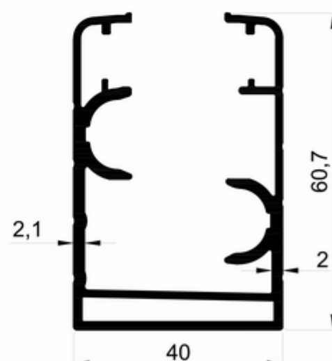
T 2529 - 1.185 kg/m
