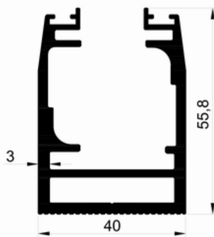
T 2254 - 1.545 kg/m
