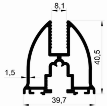
T 2563 - 0.900 kg/m
