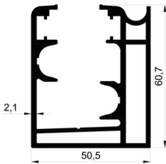
T 876 - 1.887 kg/m
