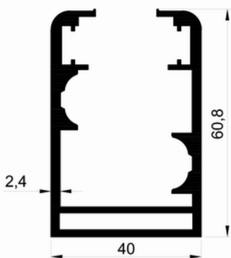
T 2425 - 1.440 kg/m
