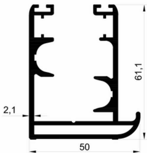
T 1073 - 1.810 kg/m
