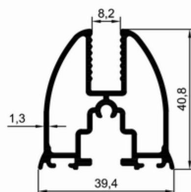
T 2564 0.840 kg/m
