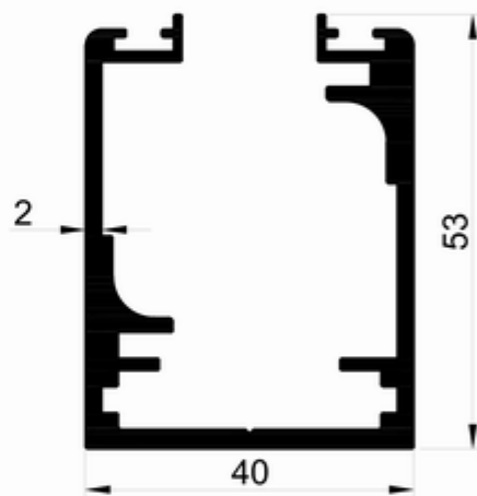
T 2160 - 1.247 kg/m
