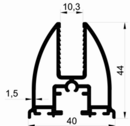
T 2533 0.990 kg/m
