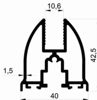
T 2534 0.919kg/m
