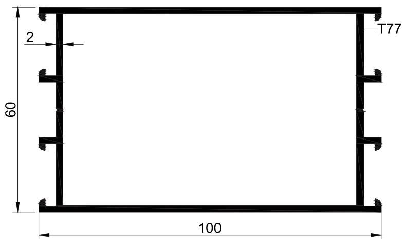
C60 T 04 -1.5mm.-1.470 kg/mt C60 T 04 -2.0mm.-1.888 kg/mt
