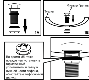
Рис 1. Монтаж плоского сифона для раковин
