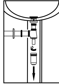
Şekil 3. Taşlı Sifon Temizliği
