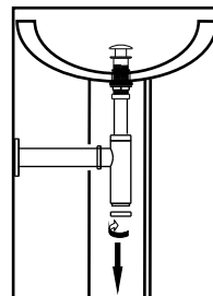
Figure 4. Nettoyage du siphon plat
