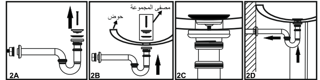
شكل 2. تركيب السيفونات بدلو و شكلU
