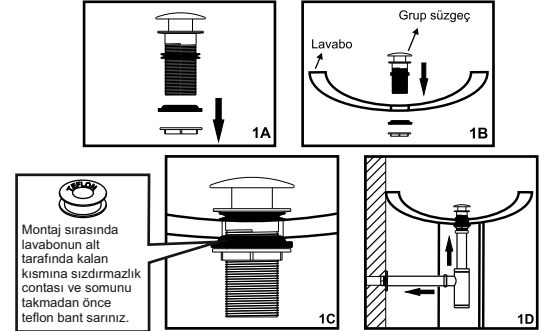
Şekil 1. Düz Lavabo Sifon Montajı
