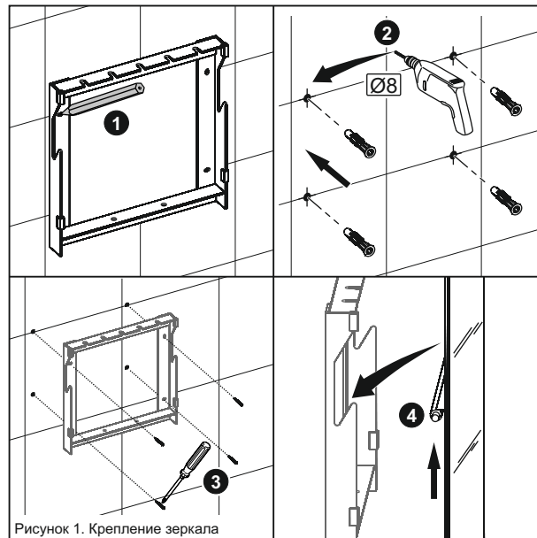
Рисунок 1. Крепление зеркала
