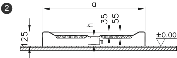
Section Kesit
